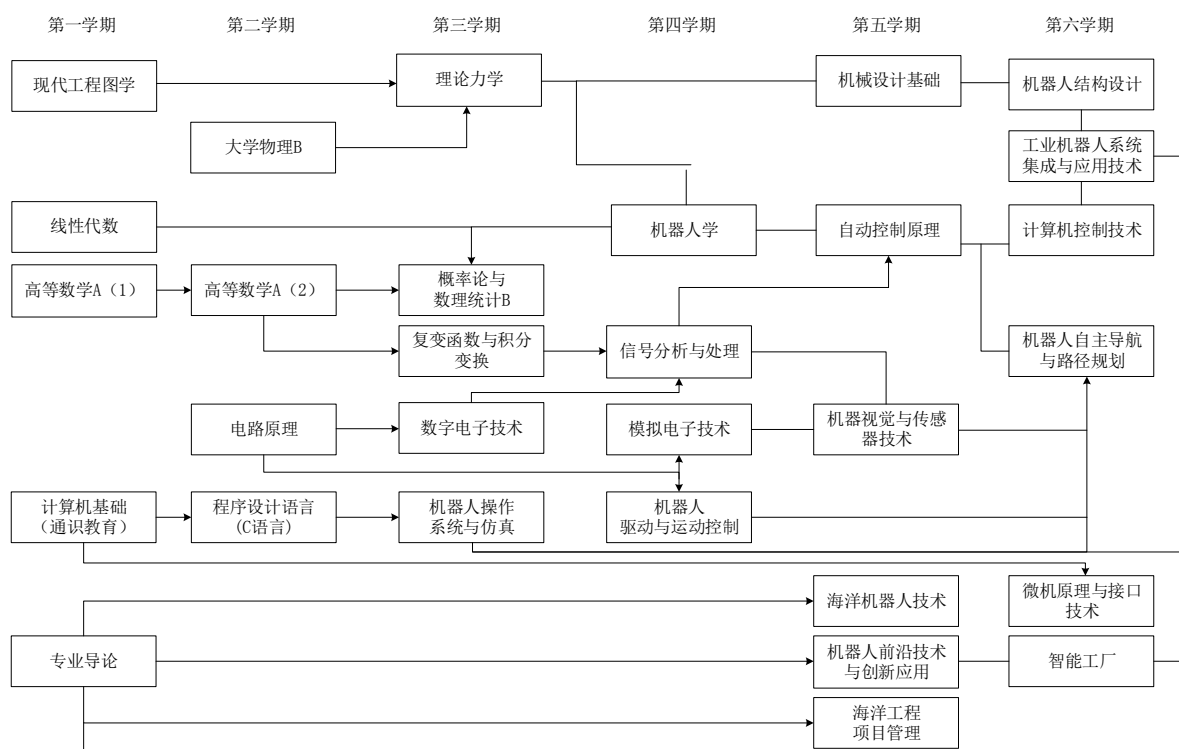
图 1 课程关系图
