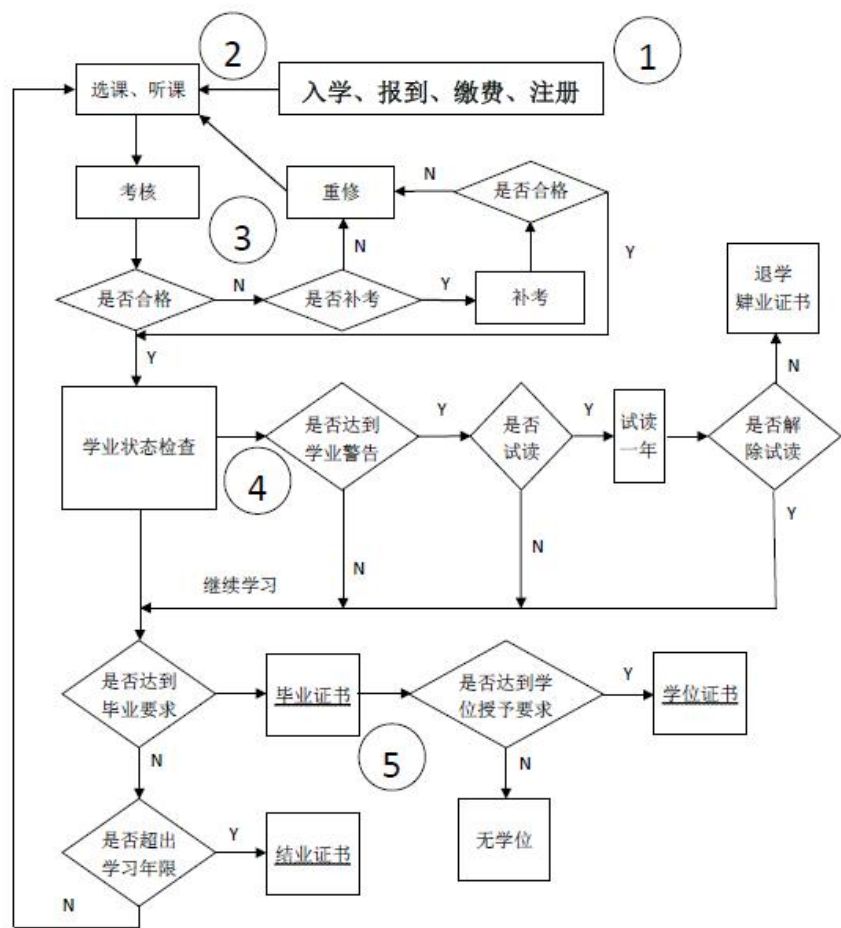
图 1 学习流程图
